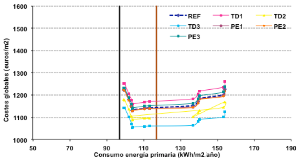
Figura 23. Análisis de sensibilidad para escenarios globales en condiciones normativas y para sistema de caldera y enfriadora y emisión convectiva.
