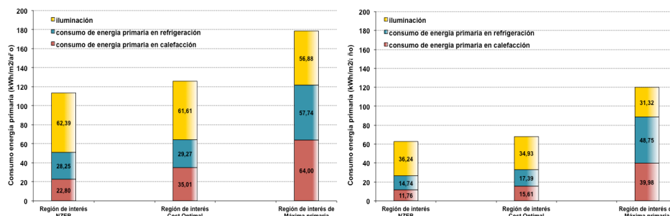
Figura 17. Distribución de consumos por usos en las regiones de interés en condiciones reales (izda.) y optimizadas (dcha.).
