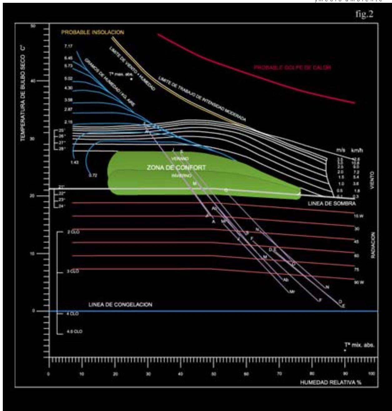
Diagrama bioclimático de Olgiay, situando las temperaturas medias de máximas y mínimas Madrid.
